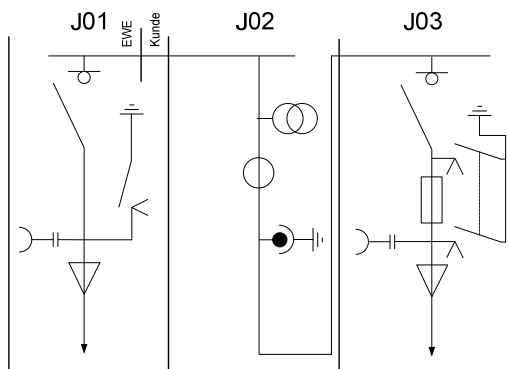
J01 ) Eingangsfeld mit Lasttrenn- und Erdungsschalter und Doppelkabelhalteisen J02 ) Feld für Zählung J03 ) Trafofeld mit Lasttrennsicherungs- und Erdungsschalter
