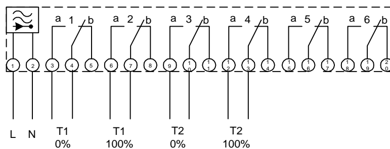
Bild 1: Schaltbild TRE
