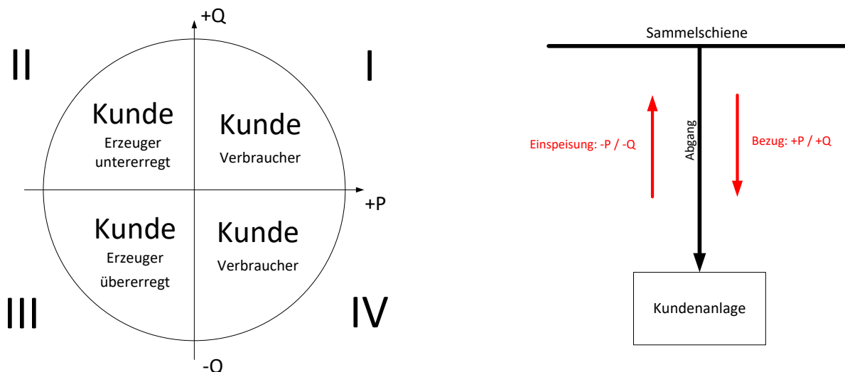
Abbildung 5: Verbraucherzählpfeilsystem – Bezugspunkt Sammelschiene am NAP
