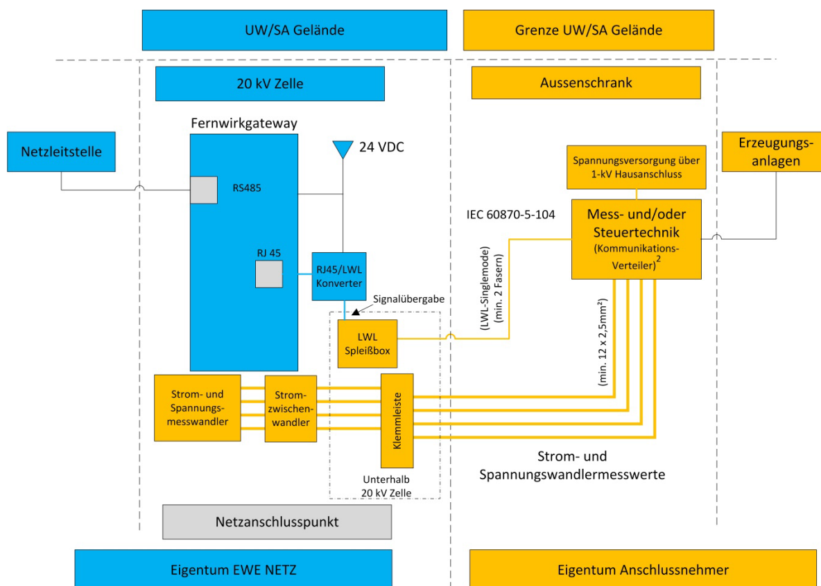
Abbildung 2: IEC 60870-5-104 Anbindung UW/SA Direktanschluss
