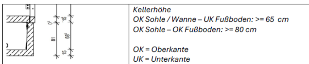
Abbildung 1: Kellermaße
