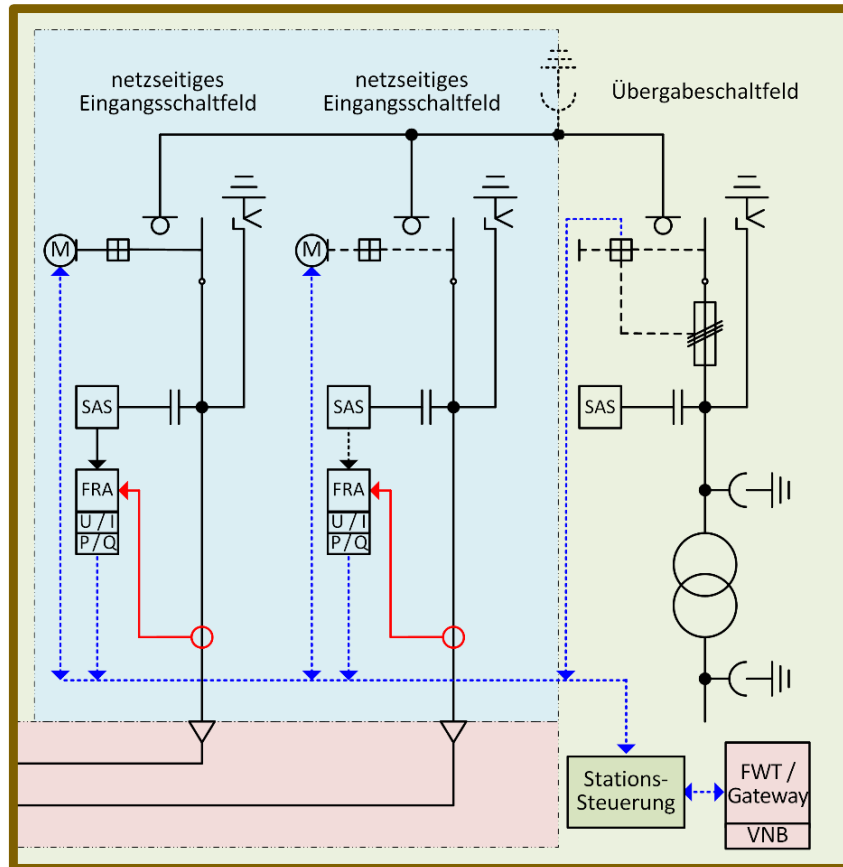
Bild D6 - KK-T – Niederspannungsseitige Abrechnungsmessung
