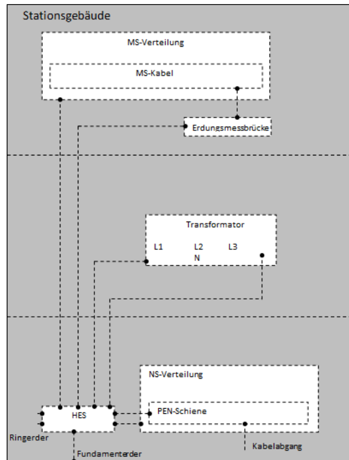
Abbildung 2: Stationsgebäude mit Erdungsmessbrücke
