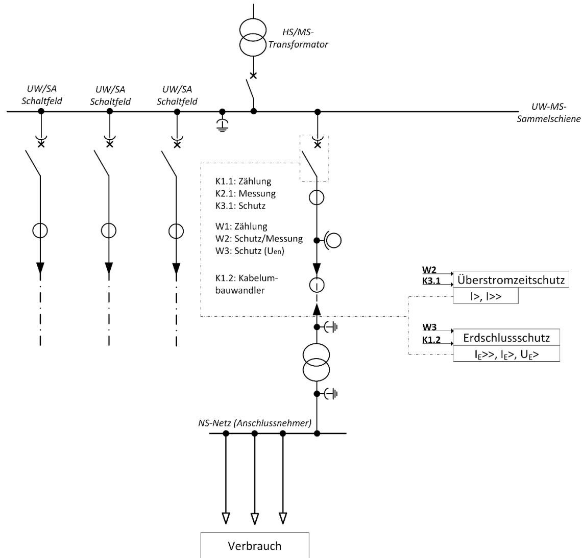
Bild D7a – Schutzkonzept für Bezugsanlagen mit Direktanschluss an ein Umspannwerk oder eine Schaltstation
