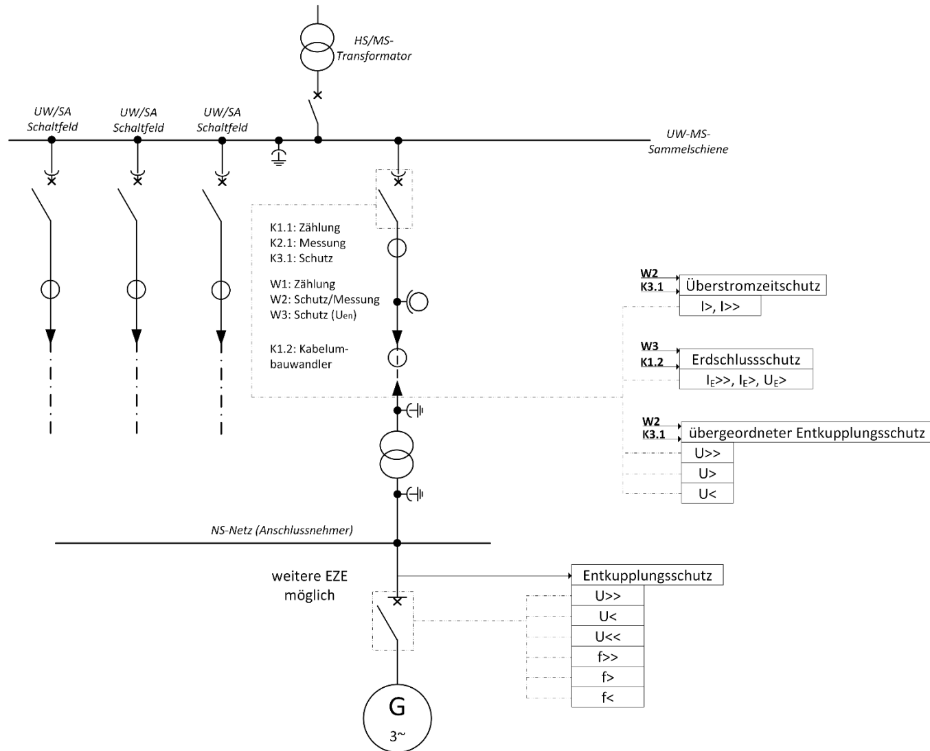
Bild D7b – Schutzkonzept für Erzeugungsanlagen und Speicher mit Direktanschluss an ein Umspannwerk oder eine Schaltstation
