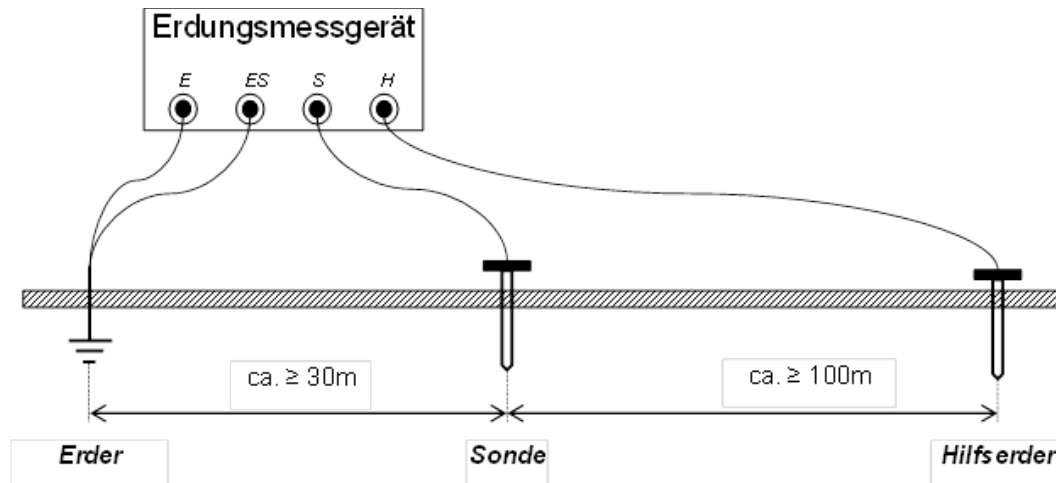
Abbildung 3: Erdungsmessgerät
