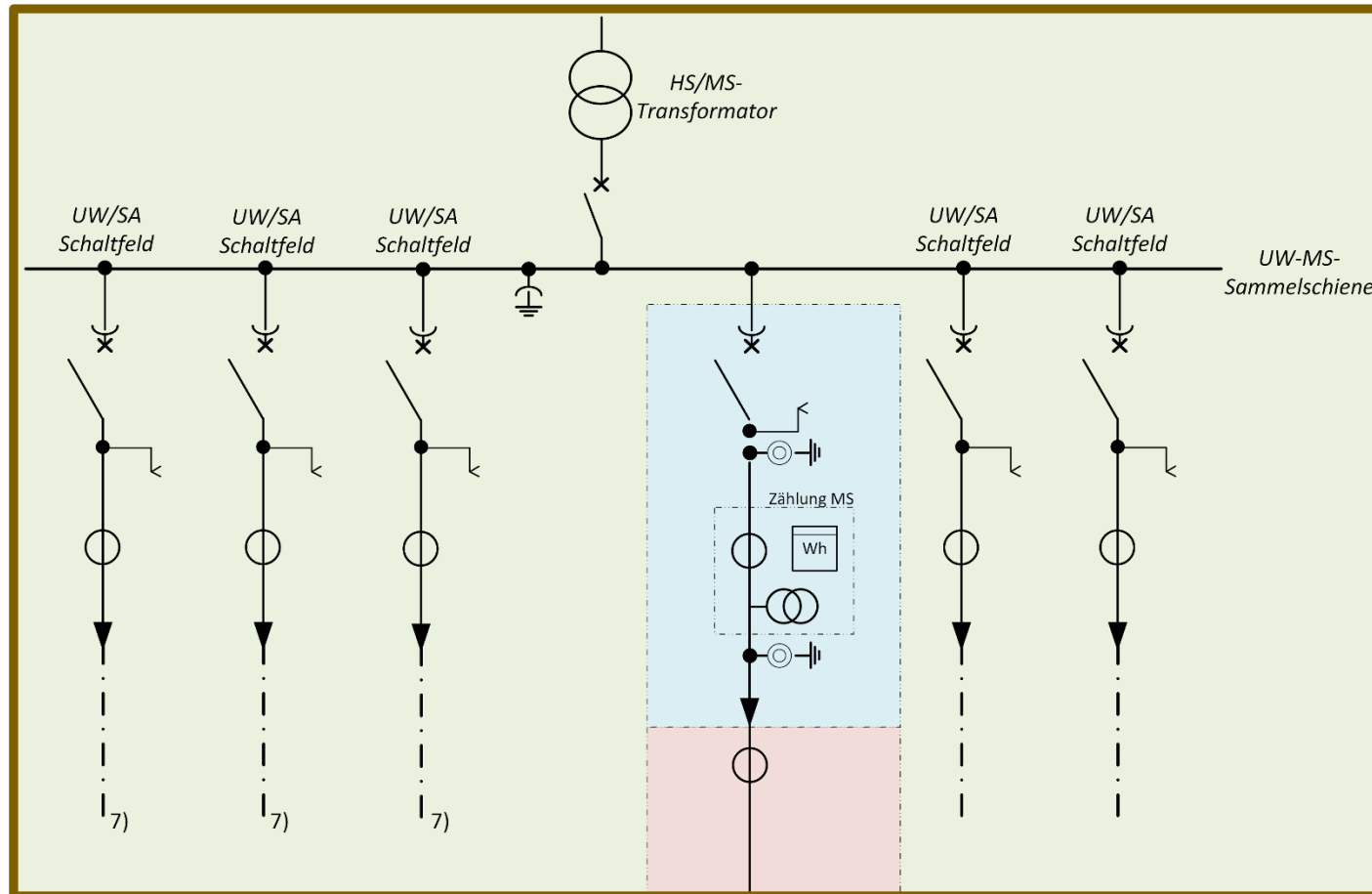
Bild D7 – Direktanschluss an ein Umspannwerk oder eine Schaltstation
