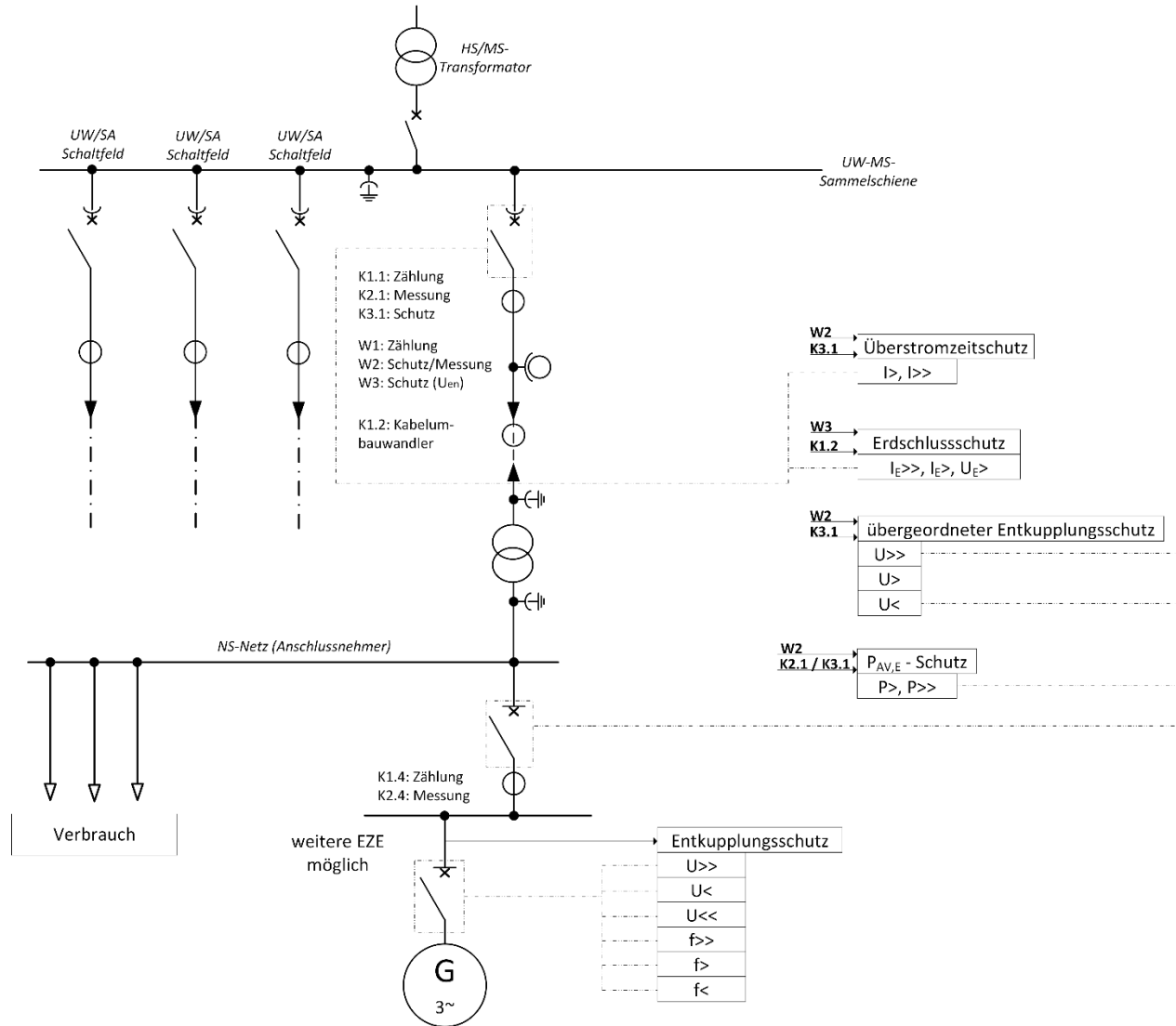
Bild D7c – Schutzkonzept für Mischanlagen mit Bezug mit Direktanschluss an ein Umspannwerk oder eine Schaltstation
