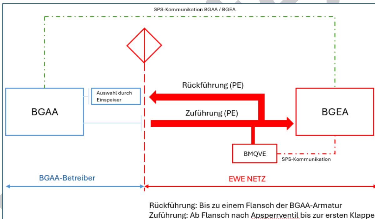
Abbildung: Darstellung der Schnittstelle BGAA / BGEA mit Biomethan-Mess-Qualitäts-Vorrichtung (BMQVE) und Probenentnahmesonde (PES)
